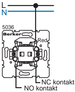
Nupplülitid (üMBERLÜLITUV kontakt)
