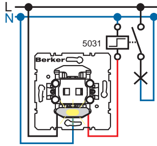
Nupplülitid (NO kontakt) Märkvalgusega (paralleelselt tohib ühendada piiramatult hulga nupplülitid) NB! Eemalda ühendussild neonlambilt
