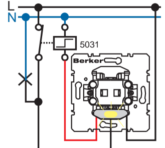
Nupplülitid (NO kontakt) (Neonlamp põleb kui valgusti on sisselülitatud) NB! Eemalda ühendussild neonlambilt
