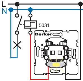
Nupplülitid (NO kontakt) Märkvalgusega (paralleelselt tohib ühendada piiratud arvu nupplülitid või kasutada neutraaljuhet)
