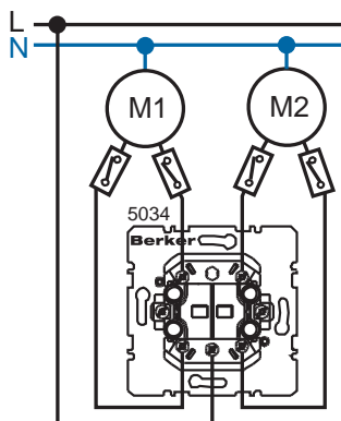
Grupinupplülitid (4 NO kontakti, ühine sisend)
