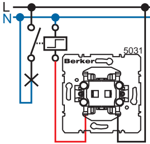
Nupplülitid (NO kontakt)
