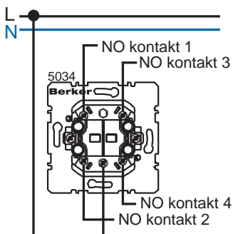
Grupinupplülitid (4 NO kontakti, ühine sisend)
