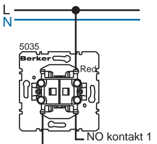
Grupinupplülitid (2 NO kontakti, ühine sisend)
