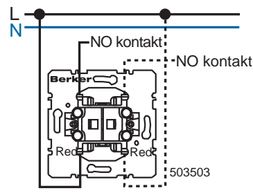
Grupinupplülitid (2 NO kontakti, eraldi sisendid)
