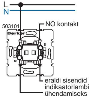
Nupplülitid (NO kontakt) eraldi sisendid indikaatorlampi ühendamiseks
