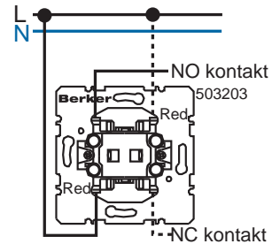
Nupplülitid (NO ja NC eraldi kontaktid)
