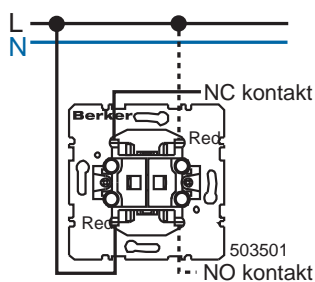
Grupinupplülitid (NC ja NO kontakt, eraldi sisendid)
