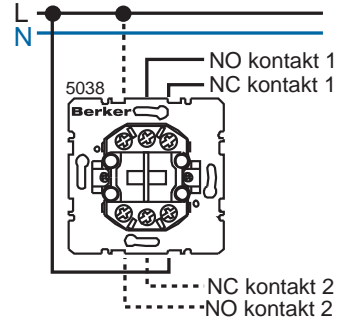
Grupinupplülitid (2 üMBERLÜLITUV kontakti, eraldi sisendid)
